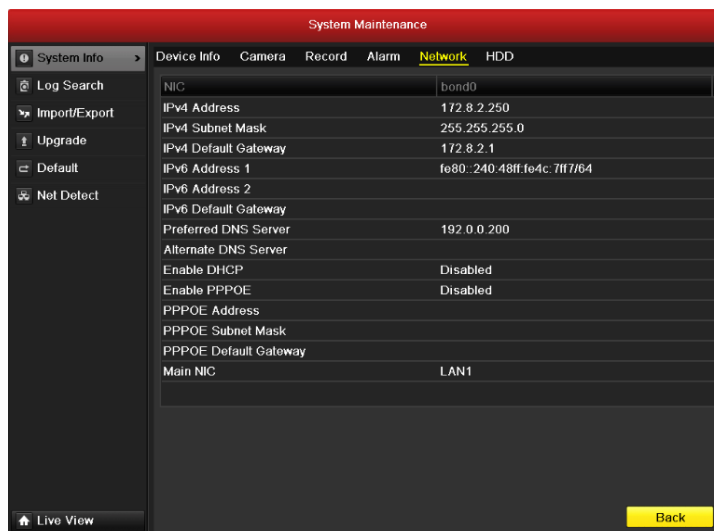
Рисунок 12.5 Интерфейс сетевой информации
