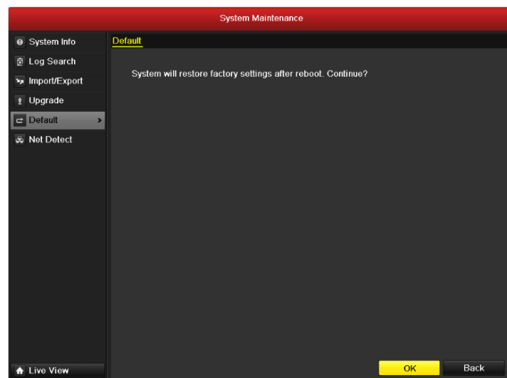
Рисунок 12.14 Восстановление заводских параметров
