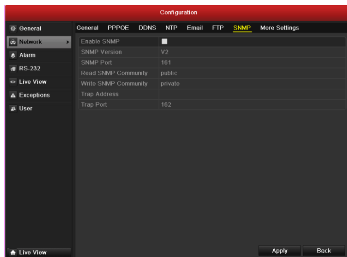
Рисунок 9.12 Интерфейс конфигурации SNMP
