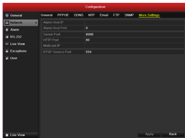
Рисунок 9.14 Интерфейс дополнительных настроек
