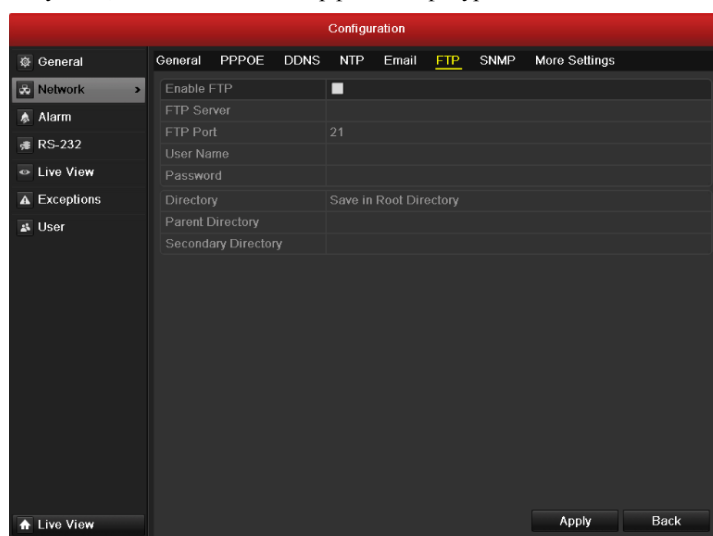
Рисунок 9.10 Интерфейс конфигурации FTP
