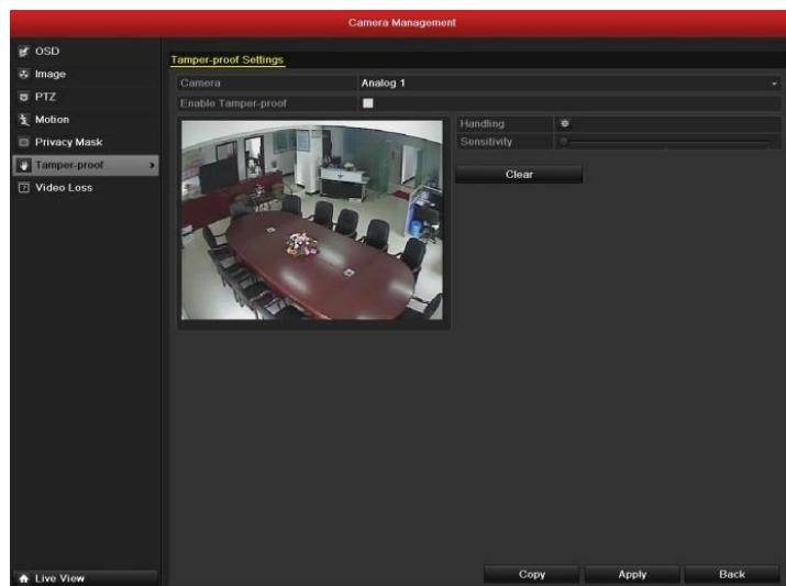
Рисунок 8.15 Интерфейс настройки детекции заслона обзора
