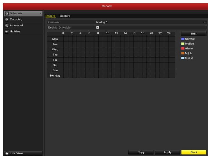
Рис 5.7 Раздел меню Record Schedule (Запись по расписанию)
