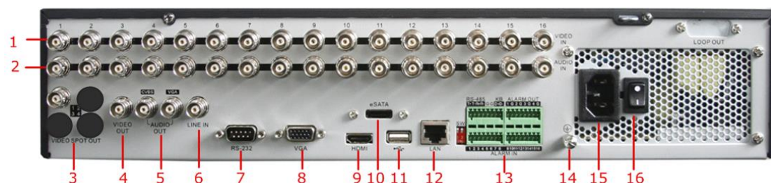
Рисунок 1.8 Задняя панель DS-8116HDI-ST
