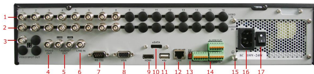
Рисунок 1.7 Задняя панель DS-8100HDI-ST
