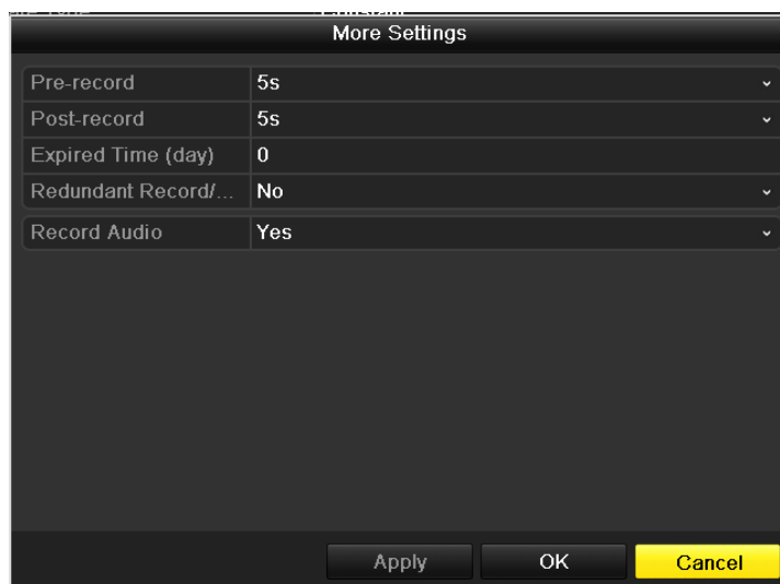
Рис 5.34 Раздел меню Encoding Record- More
