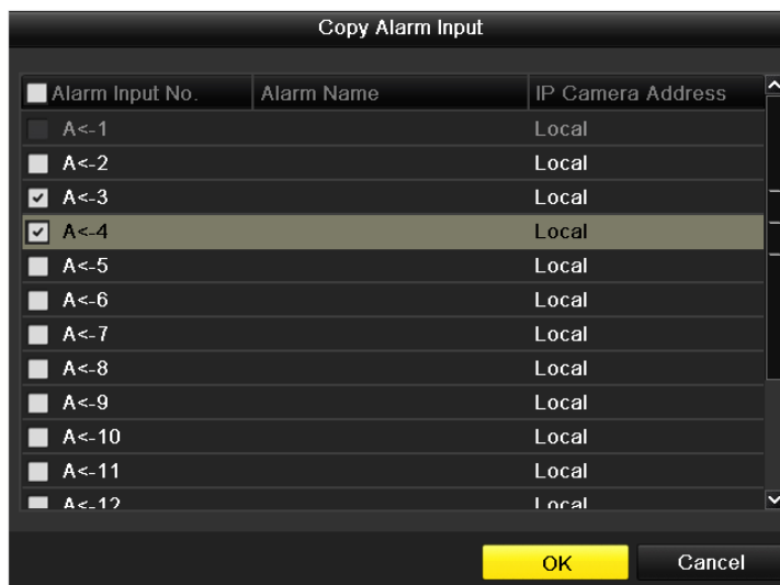
Рис 5.22 Копирование настроек тревоги
