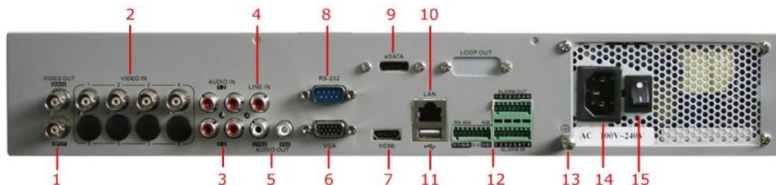
Рисунок 1.5 Задняя панель DS-7304HI-ST и DS-7304HFI-ST
