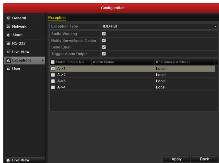
Рисунок 10.23 Конфигурация тревоги ошибок HDD
