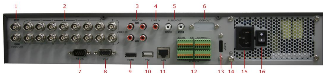
Рисунок 1.6 Задняя панель DS-7316HI-ST&DS-7316HFI-ST
