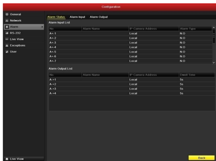
Рисунок 8.6 Интерфейс статуса тревог меню системной конфигурации
