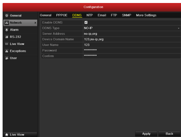
Рисунок 9.8 Интерфейс конфигурации NO-IP
