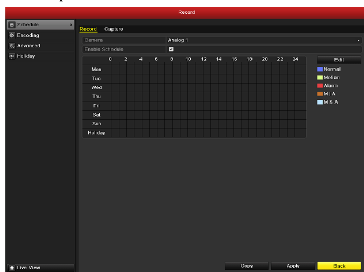
Рис 5.29 Раздел меню Record Schedule – расписание записи
